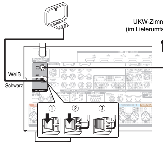
MW-Rahmenantenne (im Lieferumfang enthalten)
