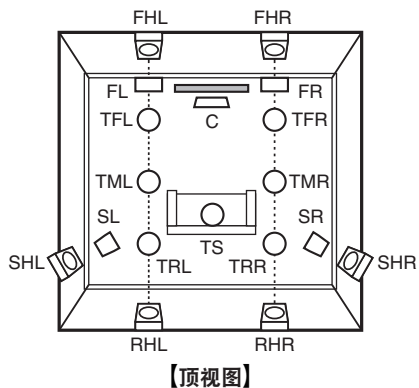
纵向扬声器布局
