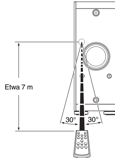
[Vertikale Aufstellung]
