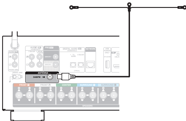
DAB-/UKW-Zimmerantenne (im Lieferumfang enthalten)
