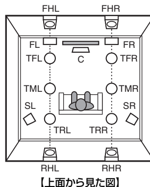
ハイトスピーカーのレイアウト図
