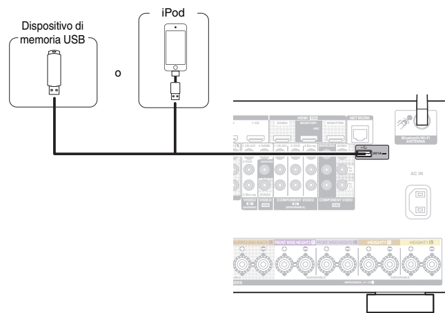
【Pannello posteriore】
