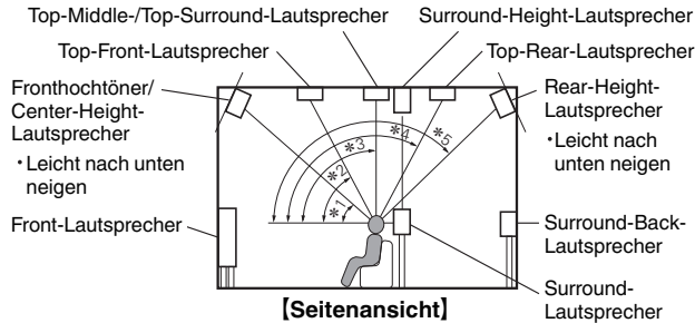
[Seitenansicht]
